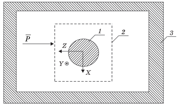
Рис. 3. Горизонтальное сечение расчетной области — плоскость XOZ (см. рис. 1); 1 — золотой наночилиндр; 2 — замкнутая поверхность, на которой было рассчитано распределение напряженности электрического и магнитного полей; 3 — АП-слой (вектор Пойтинга \vec{P} перпендикулярен оси наночилиндра)
